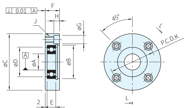
斷面 L-L
